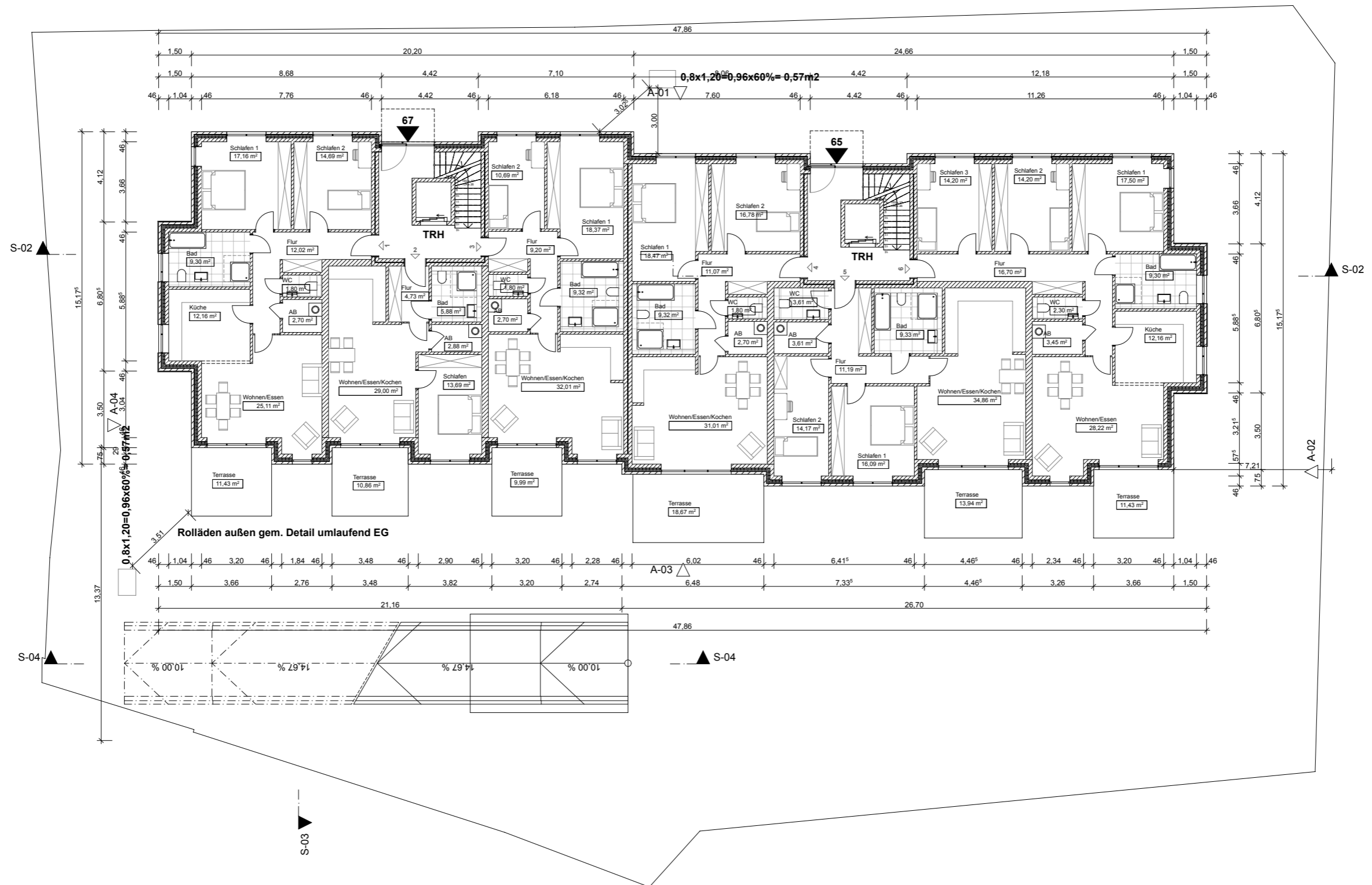
GRUNDRISS ERDGESCHOSS M 1:200
