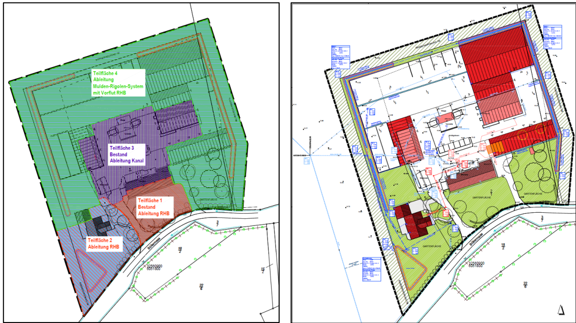
Übersicht Entwässerungsziele
