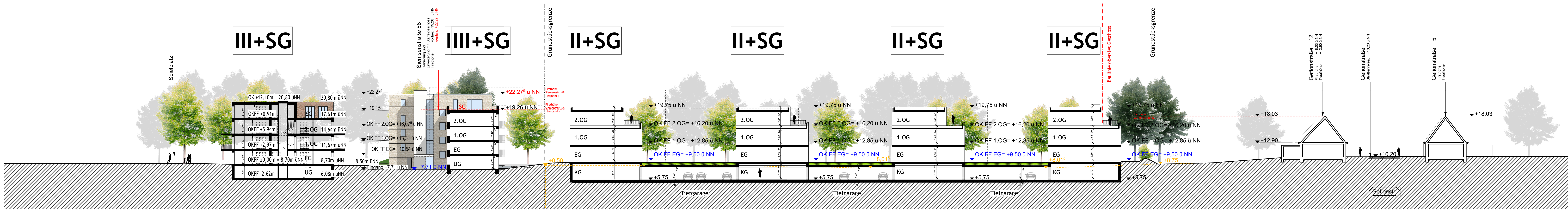
SCHNITT B-B
