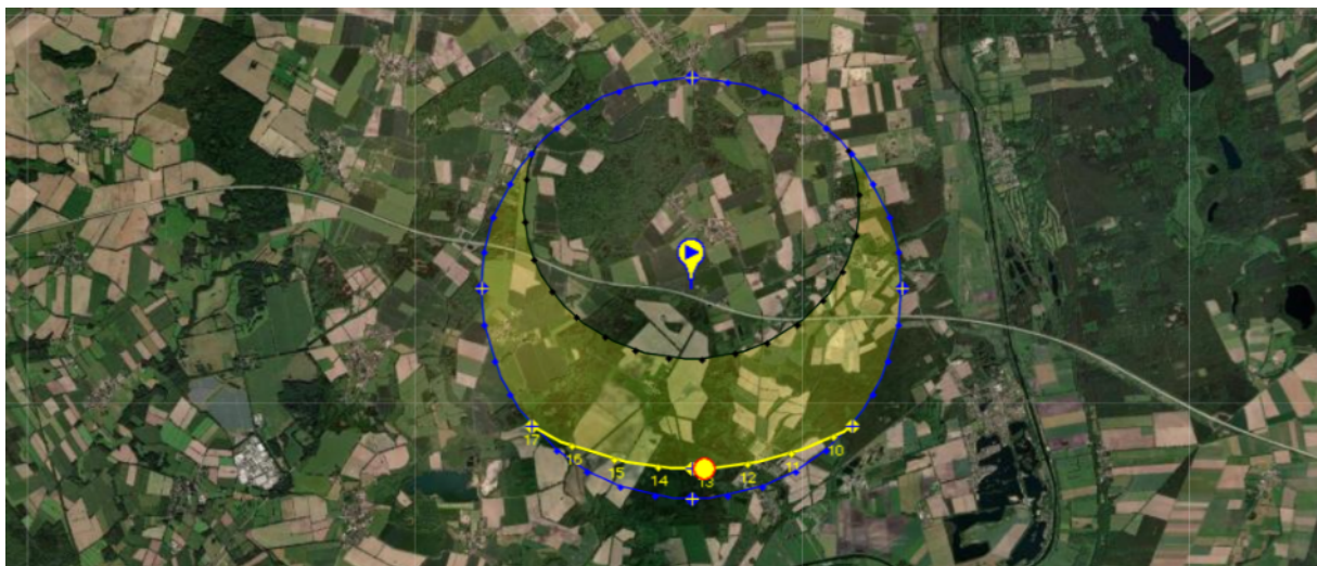
Abb.26: Sonnenstand 21.12.2025
