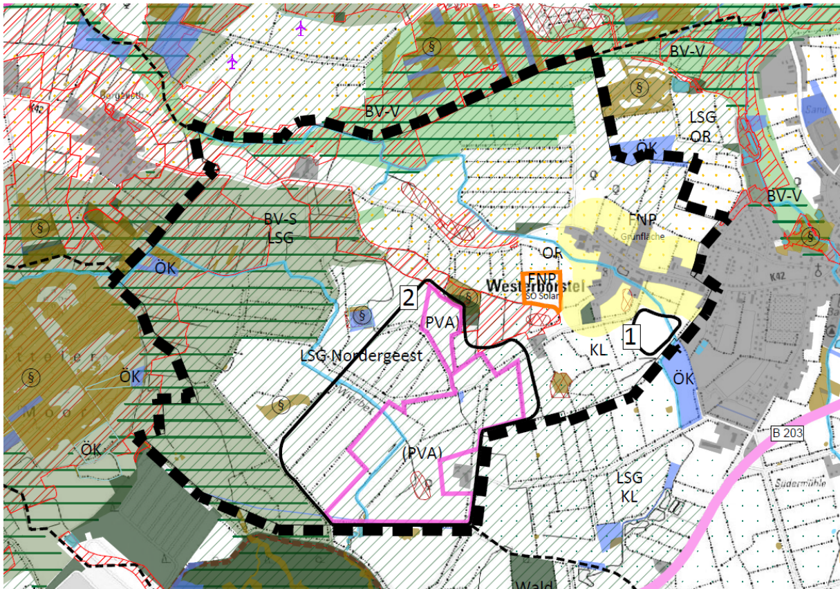
Abbildung 5 Standortkonzept, Originalmaßstab 1:15.000
