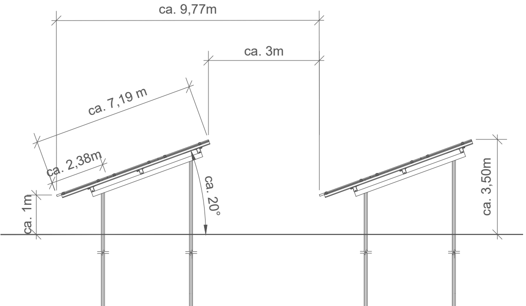
ANSICHT MODULTISCH (schematische Darstellung)
