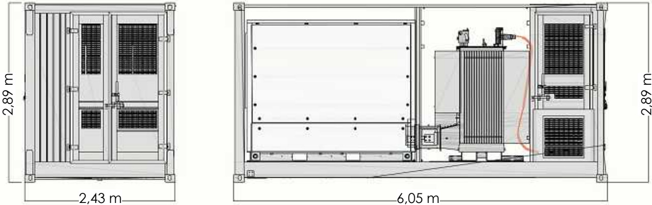
ANSICHTEN CONTAINER (MVPS) (schematische Darstellung)
