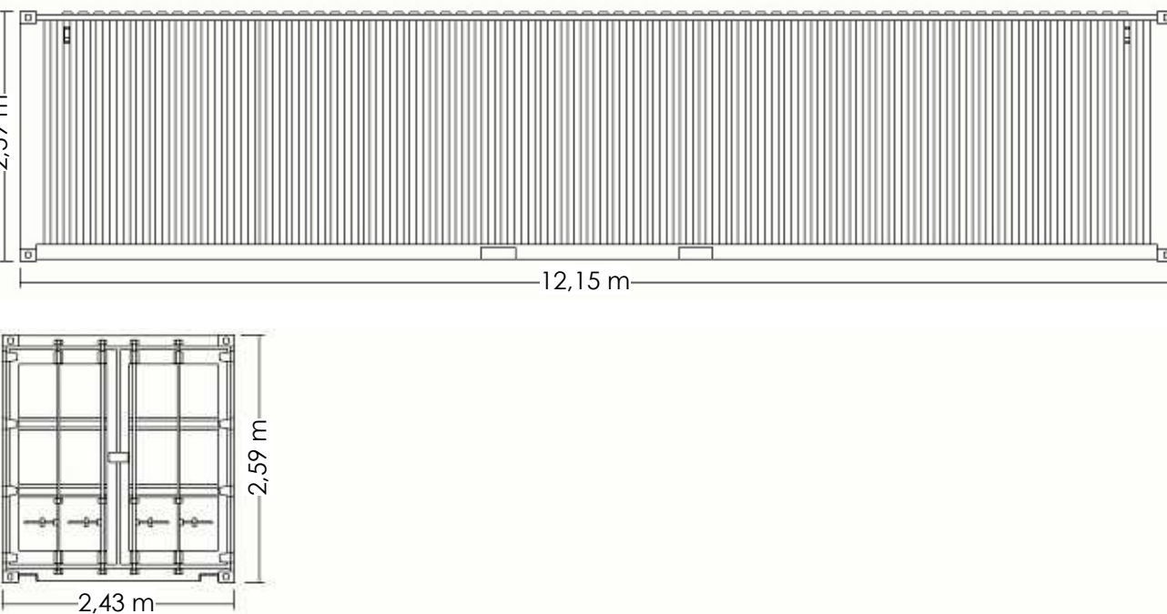
ANSICHTEN CONTAINER (Ersatzteillager) (schematische Darstellung)
