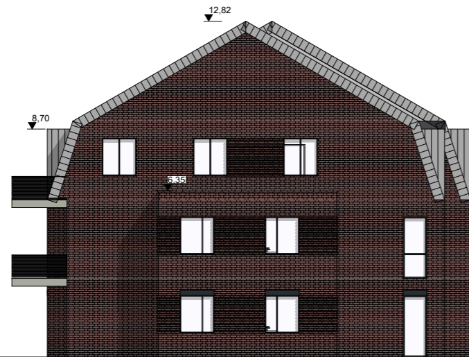
Ansicht Seite • Süd-Ost
